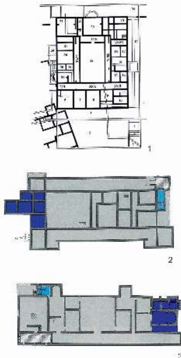
Obr. 23 Hlavné obytné budovy v rímskych vilách. 1 - stavba s vnútorným peristylom (vila Balaca v dnešnom Maďarsku), 2 - stavba s portikom a nárožnými rizalitmi (vila Müngersdorf v dnešnom Nemecku), 3 - radová stavba s chodbou a s portikom (vila Blankenheim v dnešnom Nemecku). Podľa Heimberg 2005, Abb. 27 a 30; Palágyi 2011, Abb. 2, upravil Vladimír Varsík.
